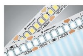
GS3503 белый 5000*10*1.2 LED 22 Вт/мW IP20 6500K холодный белый свет 2 873 р.
